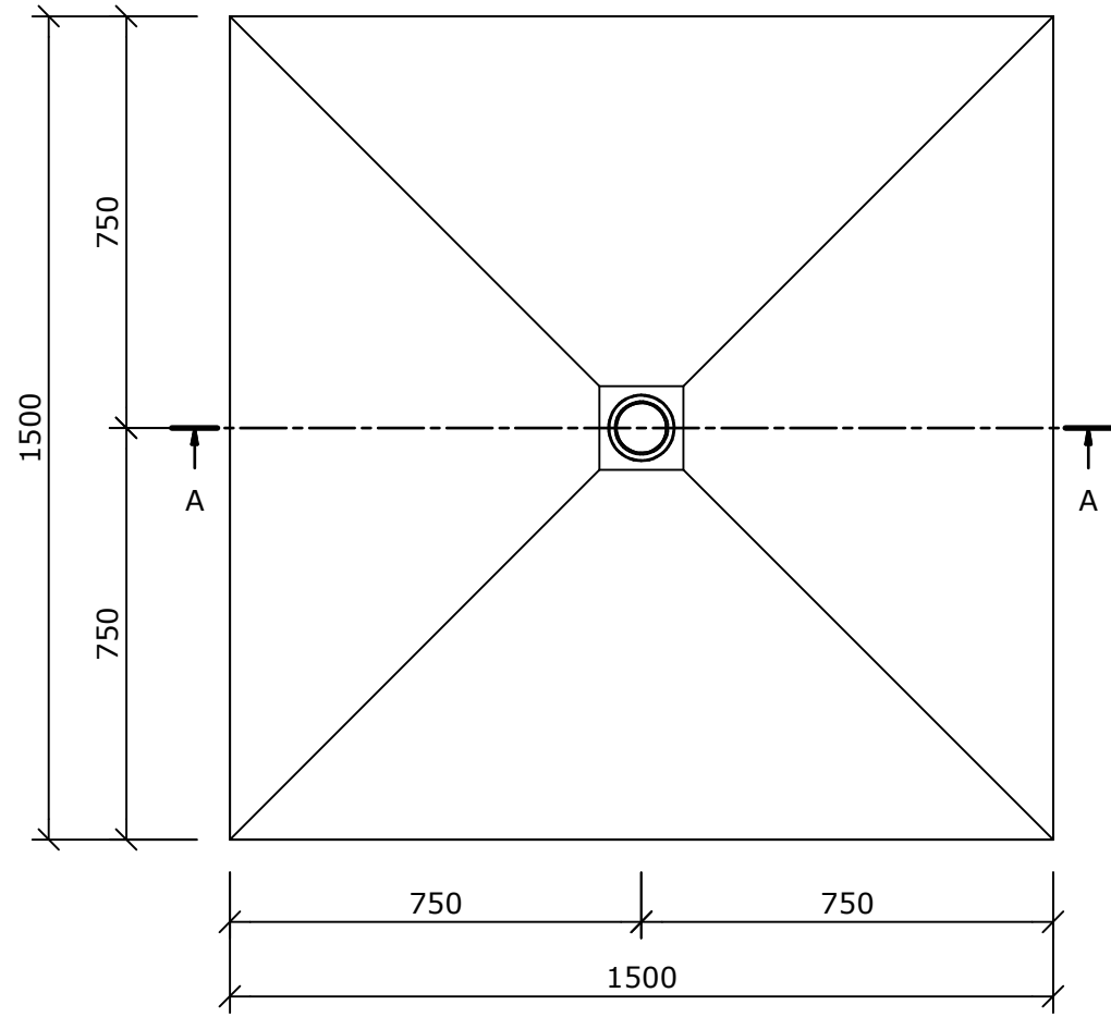
Draufsicht (1 : 15)
