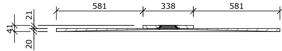
Schnitt B-B (1 : 15)
