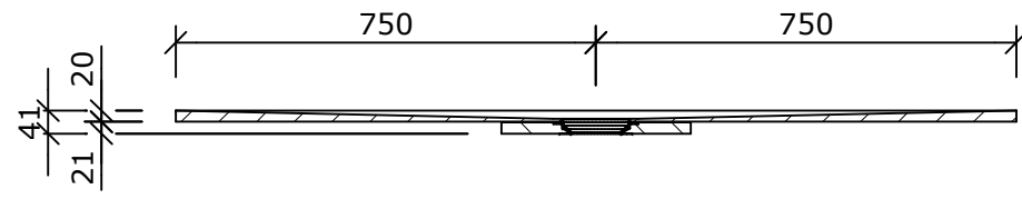
Schnitt A-A (1 : 15)
