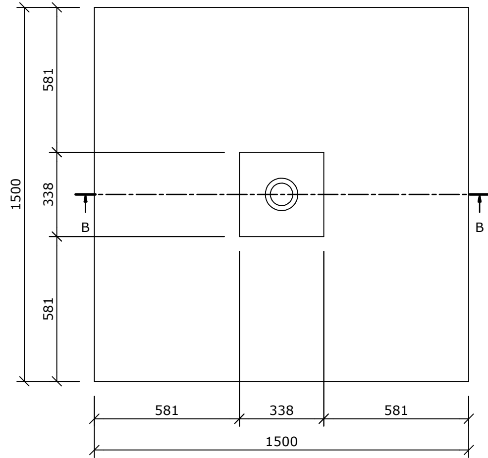
Untersicht (1 : 15)
